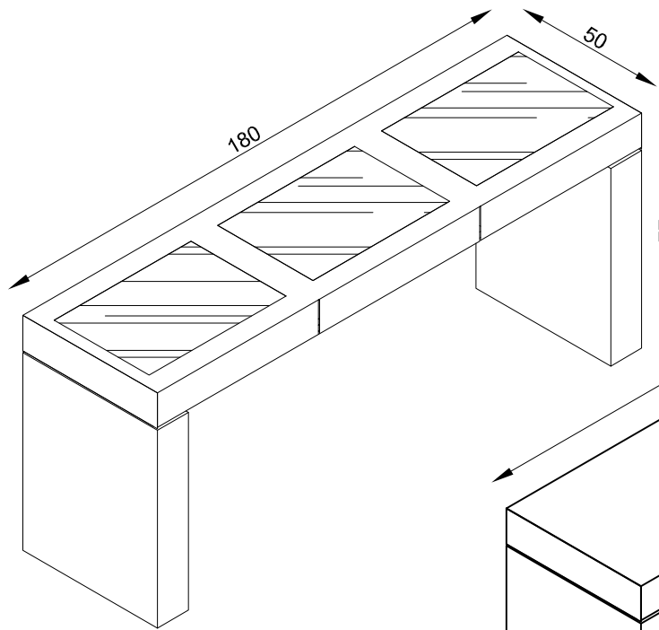
MÓDULO CISSY EM U 180CM COM RECORTE P/ VIDRO
