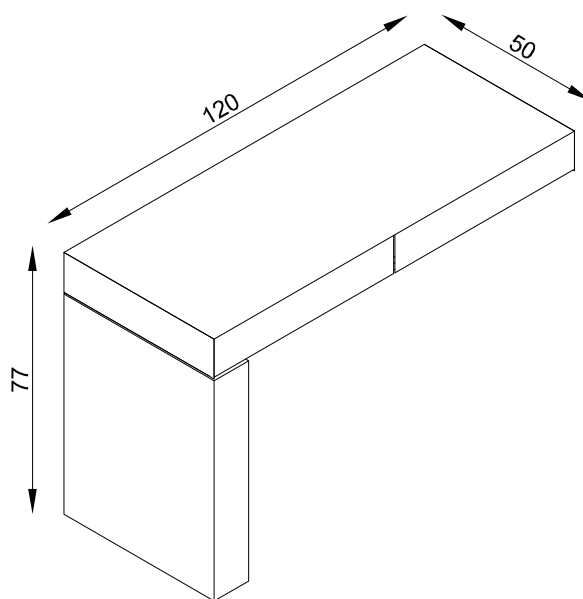
MÓDULO CISSY EM L LADO ESQUERDO 120CM SEM RECORTE P/ VIDRO
