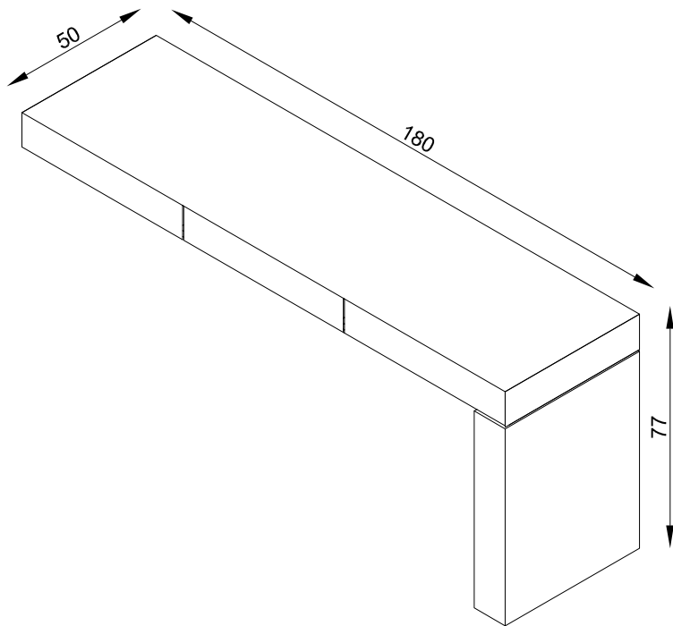
MÓDULO CISSY EM L LADO DIREITO 180CM SEM RECORTE P/ VIDRO
