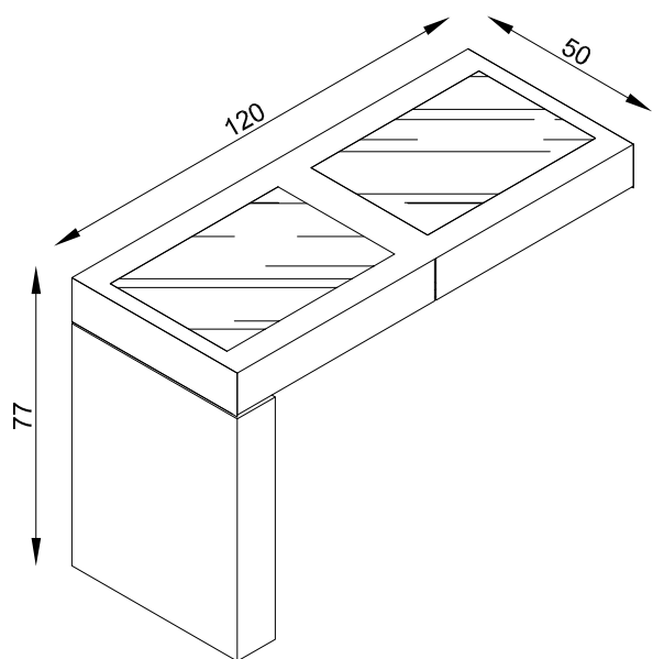
MÓDULO CISSY EM L LADO ESQUERDO 120CM COM RECORTE P/ VIDRO
