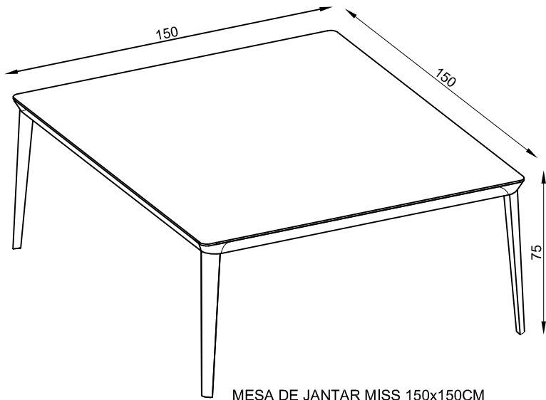
MESA DE JANTAR MISS 150x150CM
