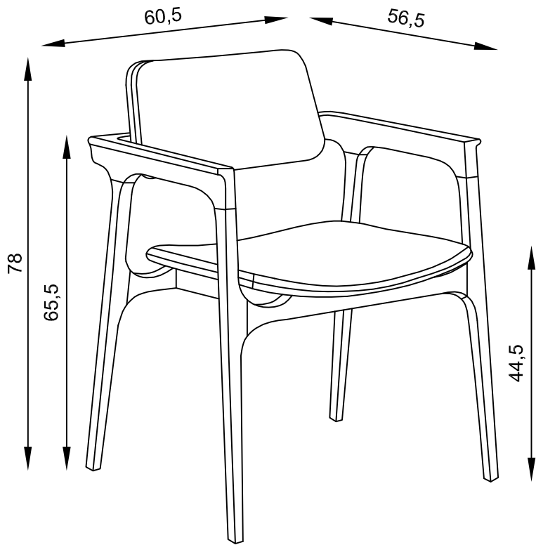
CADEIRA DITTA ESTOFADA
